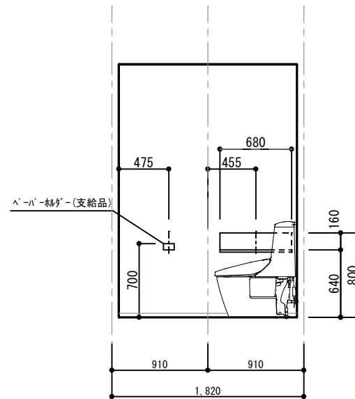
WC① 南面
