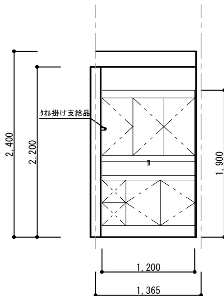
洗面 北面
