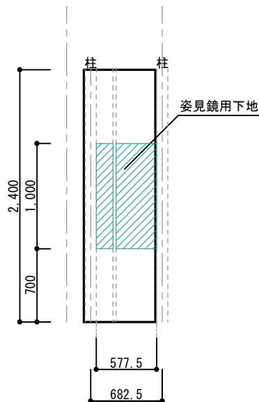
SC 西面
