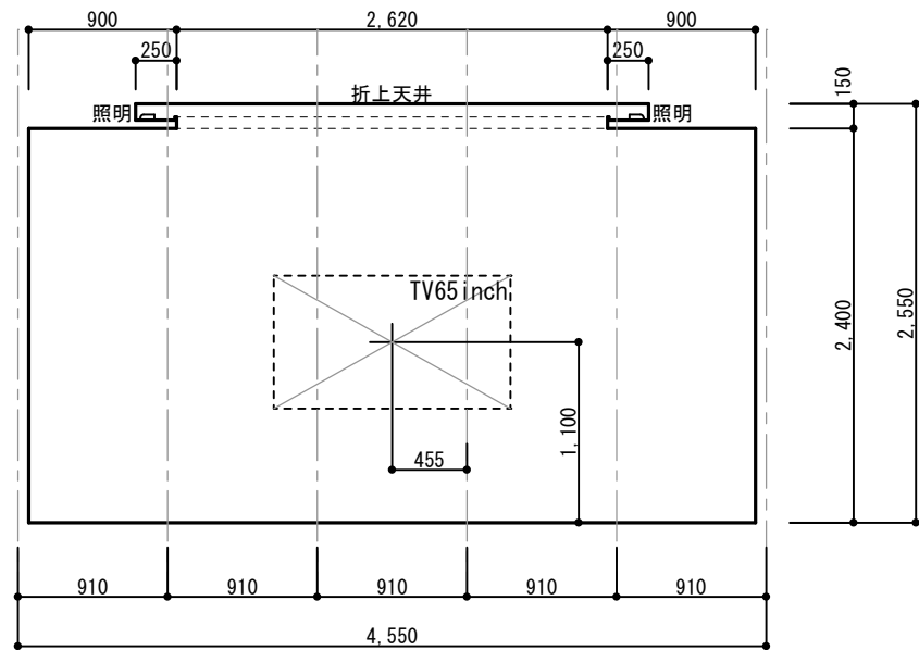
LDK① 西面
