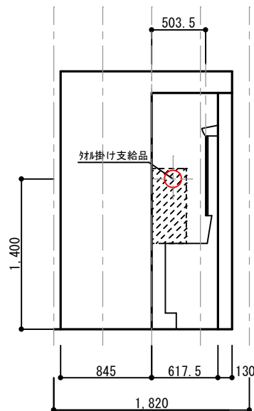
洗面 西面
